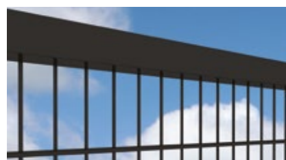
Coulissant sur rail Minerva Treillis soudés 8/6/8 mm maille 200x50 mm
